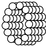
Fig.3.6g. Tubulin
