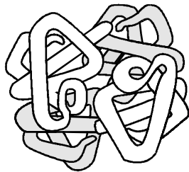
Fig.3.6d. Haemoglobin
